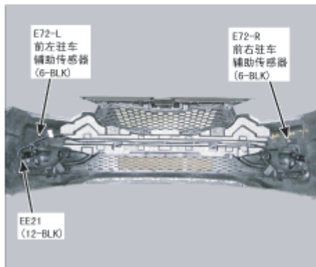
109. 前保险杠
