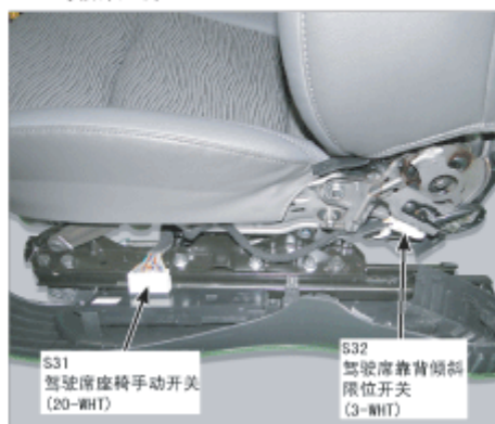
113. 驾驶席座椅
