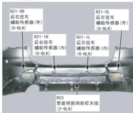
110. 后保险杠
