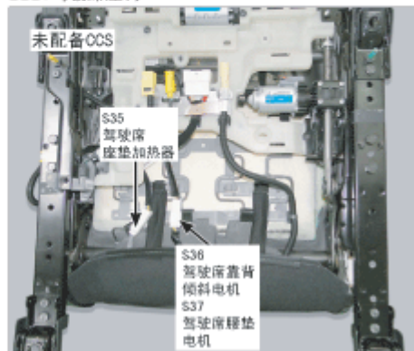
111. 驾驶席座椅
