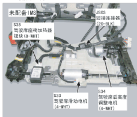
114. 驾驶席座椅
